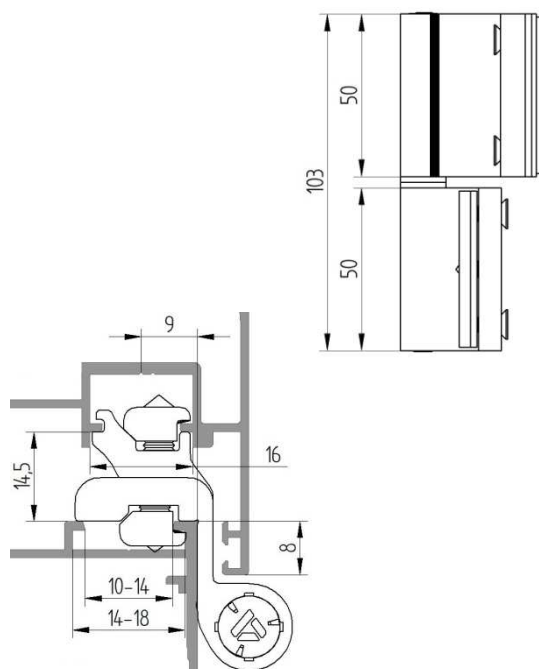
MEDIDAS Y ESQUEMA DE MONTAJE (mm.)
