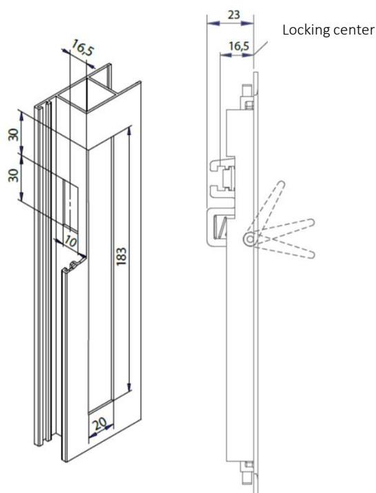
DIMENSIONS (mm.)
