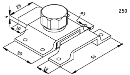
DIMENSIONS (mm.)
