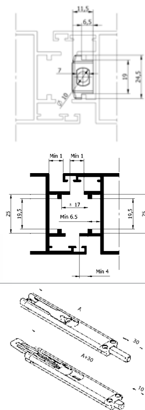
MEDIDAS (mm) Y ESQUEMA DE MONTAJE
