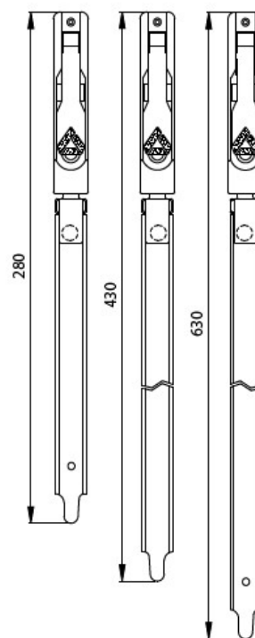
DIMENSIONS (mm.)
