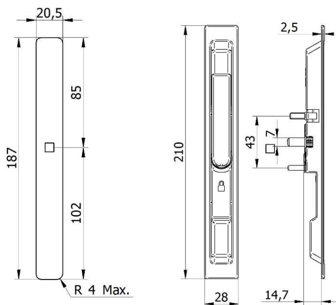
DIMENSIONS (mm.)
