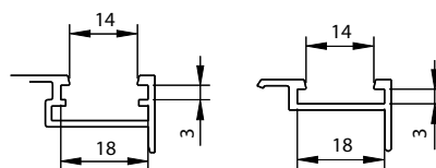
GORGES DU PROFIL INVERSEUR
