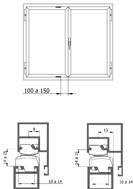
COLOCACIÓN Y ESQUEMA DE MONTAJE
