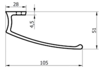
MEDIDAS (mm.) Y CENTRO DE TALACROS
