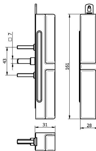
DIMENSIONS (mm.)
