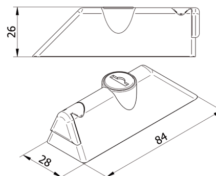
DIMENSIONS (mm.)
